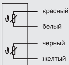
2 x Pt100, 2-проводная схема соединения
