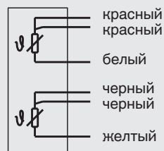
2 x Pt100, 3-проводная схема соединения
